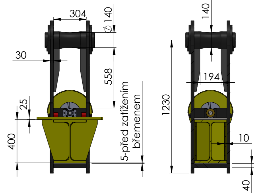
ŘEZ A-A MĚŘITKO 1 : 20
